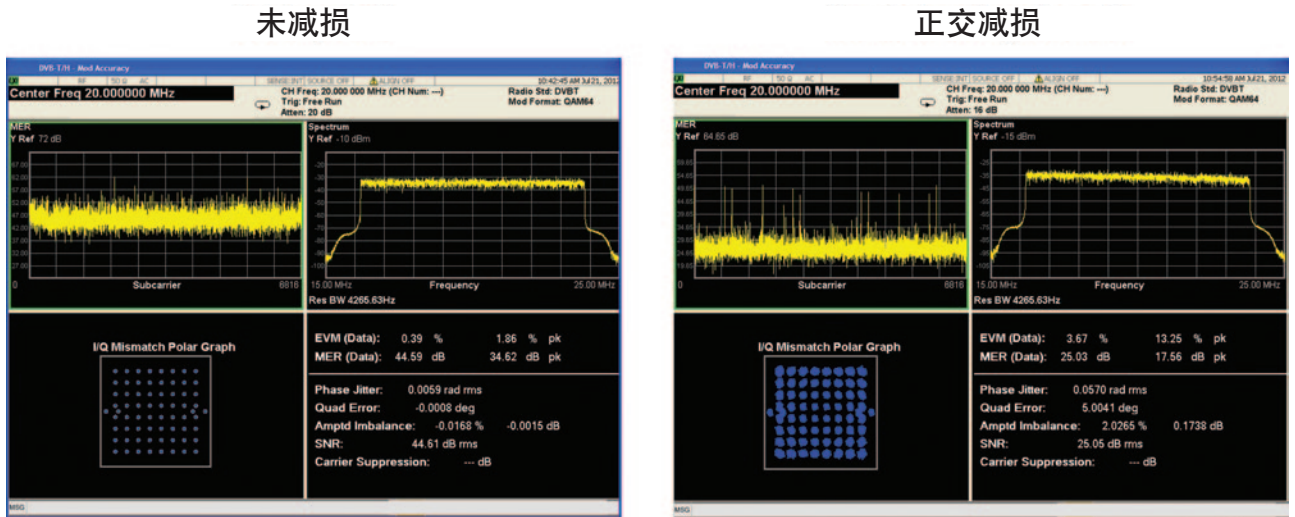
图 9. OFDM 信号生成不仅需要良好的波形发生器性能，还要使用长记录长度。DVB-T 信号(8K 模式)需要几 MSa 空间来存储至少 68 个 OFDM 符号，以便携带接收机所需的 TPS 信息，从而恰当地进行信号解调。图中，Keysight 33522B 波形发生器生成的理想信号(左图)具备出色的调制质量性能(MER > 45 db)。如右图所示，该信号是在函数发生器中，设置正交误差(5 度)和幅度失衡(2%)后输出的信号。分析仪测试结果显示了 33522B 任意波形发生器失真控制的精度。
