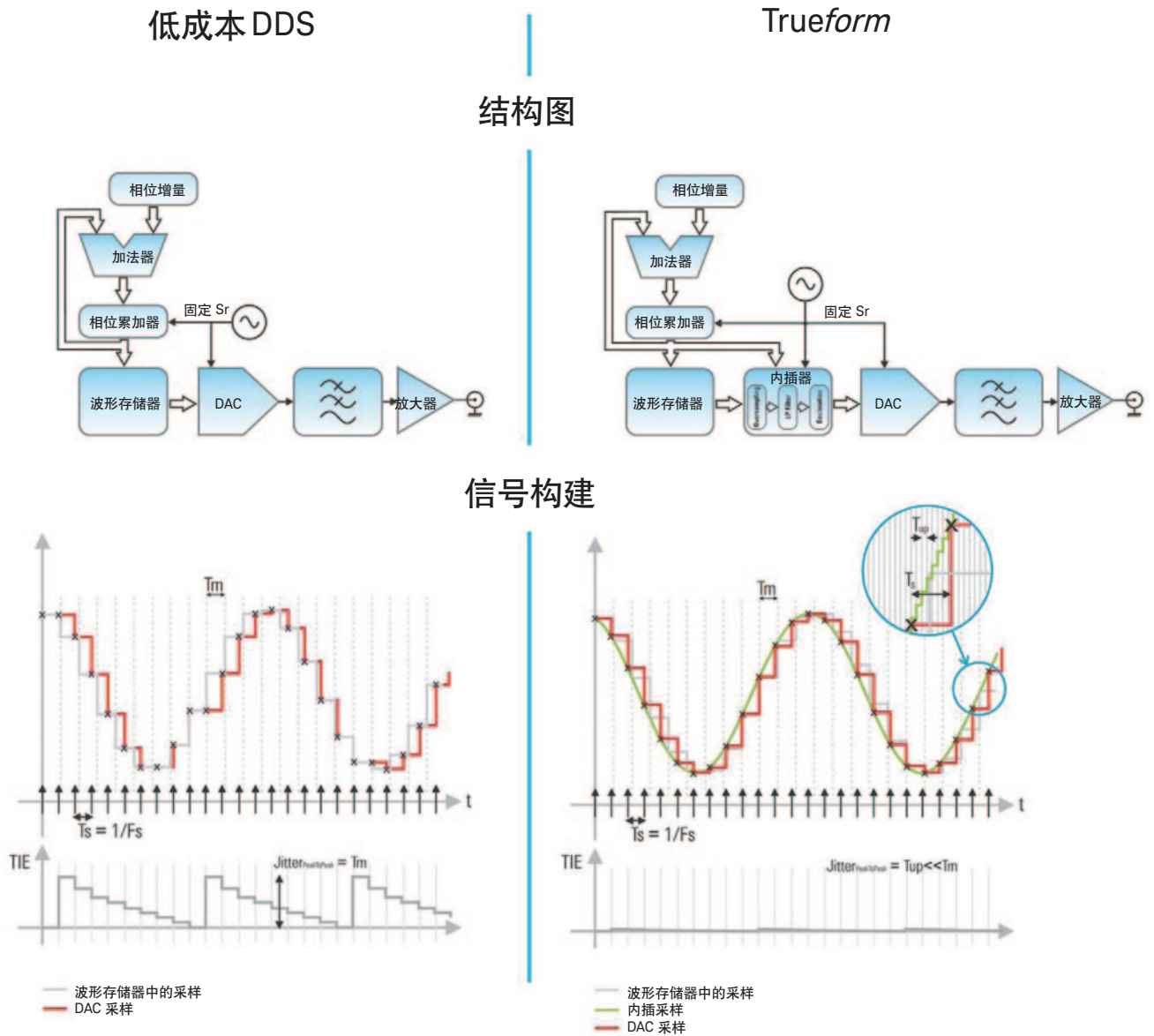
图 4. DDS 与 Keysight Trueform 技术。传统 DDS 体系结构(左图)访问波形存储器结果的方式会产生难以接受的抖动, 不利于调制信号生成。在新型 Keysight Trueform 体系结构(右图)中, 它对存储器内的信号进行实时的滤波、内插和重复采样, 从而消除了抖动。
