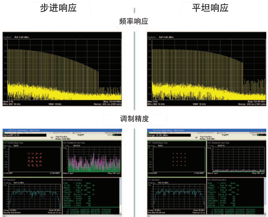
图6. Trueform 体系结构能够优化波形发生器针对平坦度或步进响应的频率响应。常规任意波形发生器通常针对步进响应进行优化。图中，在 1 MHz 至 100 MHz 频率范围内的 100 阶频信号可用于评测两种滤波器模式中的频率响应(顶部)。在两种滤波器模式下，生成一个 20MBaud 16QAM 信号并进行质量分析，显示了平坦响应特性对于高质量宽带调制生成的重要性(底部)。借助 250MHz 采样率和 Trueform 信号生成技术，可用数字带宽明显高于其它生成技术的带宽，通过使用软件对数字带宽进行归一化，在 100MHz 时，同样可以获得良好的平坦度。
