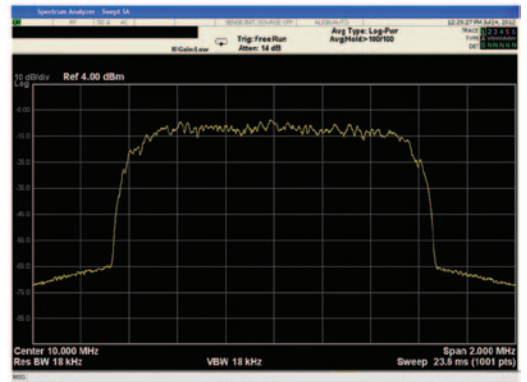
图5. DDS与Keysight Trueform技术的星座图和频谱图。图中,使用DDS和Trueform发生器生成同一个QPSK信号。两者的调制质量(EVM, 矢量幅度误差)和频谱质量相差很大(注意动态范围内的20 dB差别)。在DDS星座图中的椭圆分布点(红色)显示了抖动在调制域中作为相位噪声存在;纯噪声(高斯噪声)可使Trueform发生器的星座图点呈圆形。由DDS体系结构产生的采样抖动会导致频谱增益。
