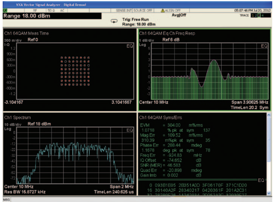
图8. 调制信号的性能体现为调制质量和频谱失真。除了模拟理想的调制信号，模拟和仿真调制信号经过传输设备或不同的传播路径等过程引起的失真在测试中也是非常重要的。在图中，就是使用Keysight 33522B波形发生器生成具有多径失真的64 QAM信号。Keysight CXA分析仪内部的自适应均衡器可以校正失真影响且显示对应的信道响应(右上方)。校正后的信号可获得非常理想的调制质量(EVM < 0.3%)。
