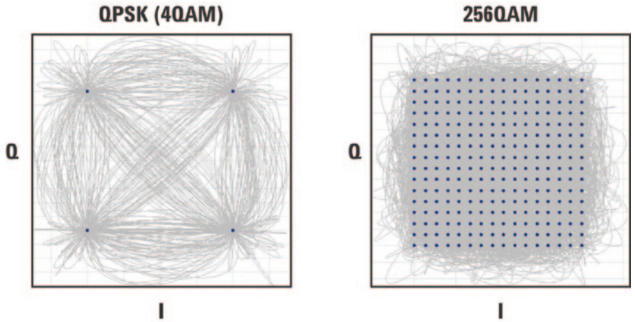
图2. 相位/星座图能够方便地显示调制方案。从根本上讲, 它们属于I/Q 笛卡尔表示, 可直接转换为针对调制载波状态的极坐标(幅度与相位)表示。图中显示了QPSK和256QAM调制的星座图(蓝点)。QPSK调制将2个比特映射为1个符码, 256QAM调制则将8个比特映射为1个符码; 对比两种调制, QPSK的不同符码位置的间距较大, 因此QPSK调制更加适应噪声大或精度要求低的系统。
