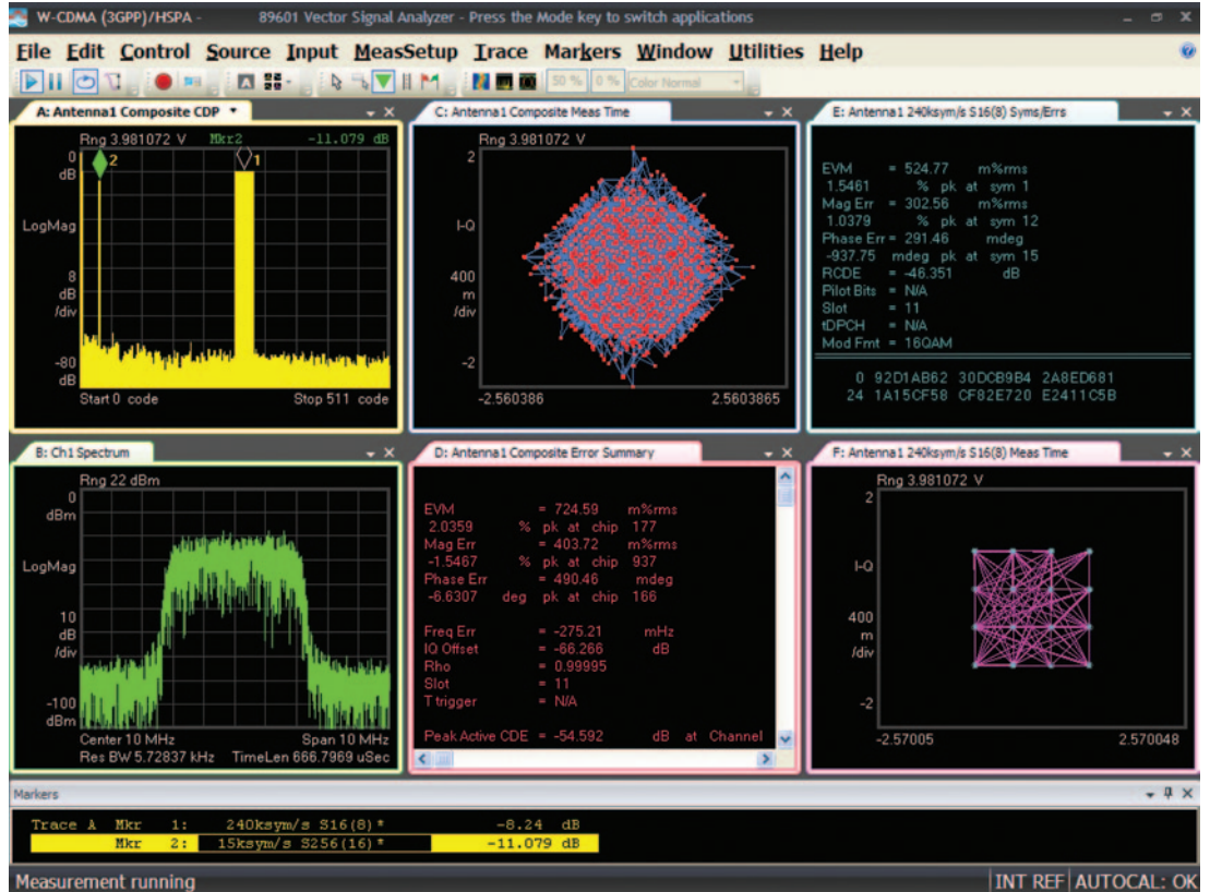
图 10. 由 Keysight 33522B 波形发生器生成的 3GPP(UMTS)WCDMA 下行链路中频信号。这是一个复杂的信号,它能够携带不同的数据和同步信道。
