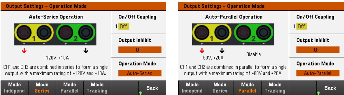
图 3. 通过自动串联和并联操作，将输出电压/电流加倍
