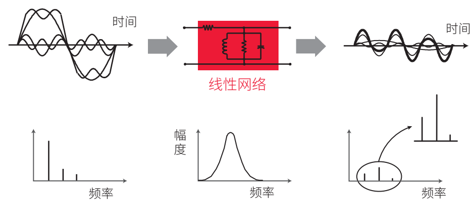
图 2. 不同频率下的幅度变化
