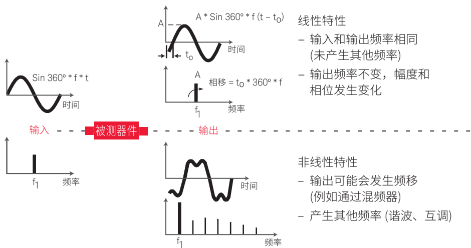
图 1. 线性与非线性特性对比
