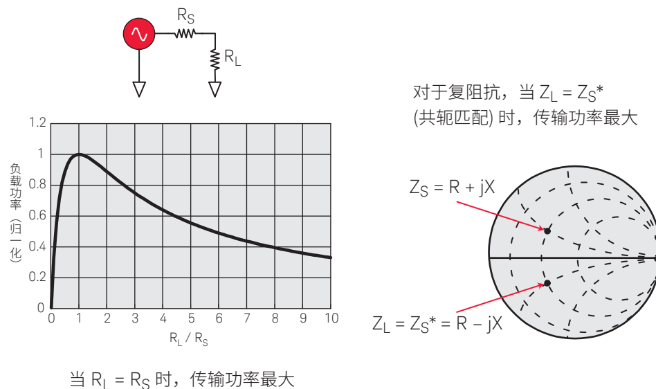
图 7. 功率传送
