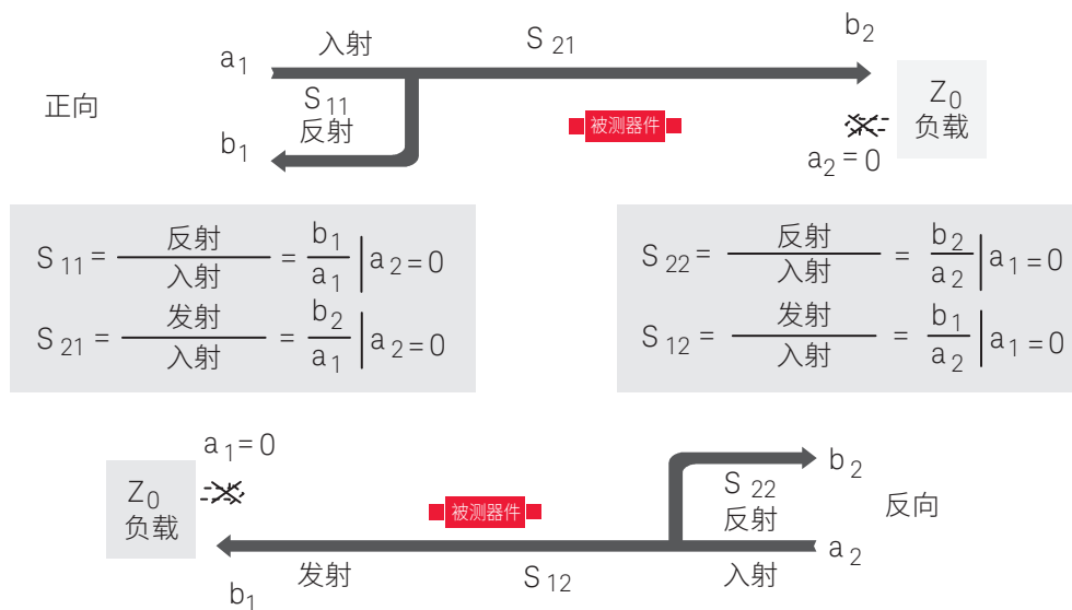
图 17. 测量 S 参数
