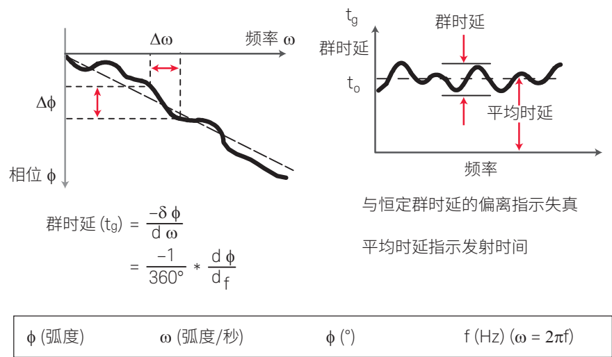
图 14. 什么是群时延?
