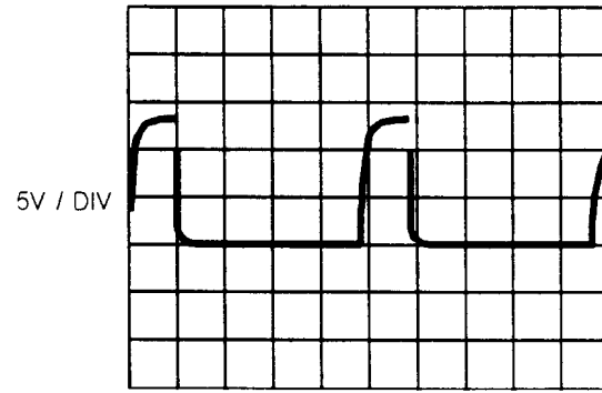
D. L201-L204, L213-216 DRIVE SIDE
