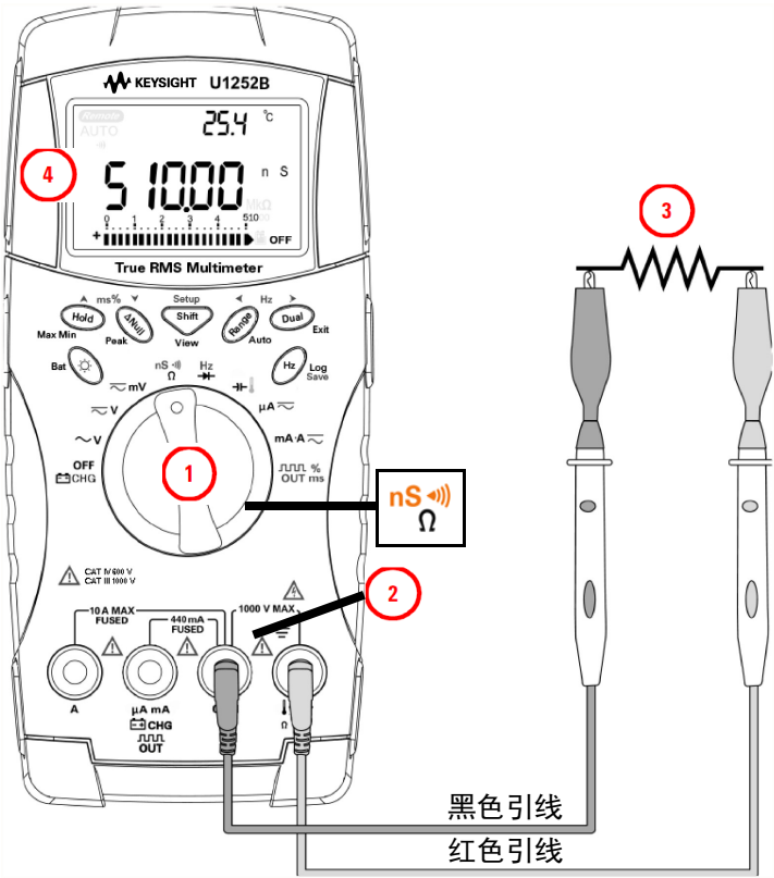
图 2-9 电导测量
