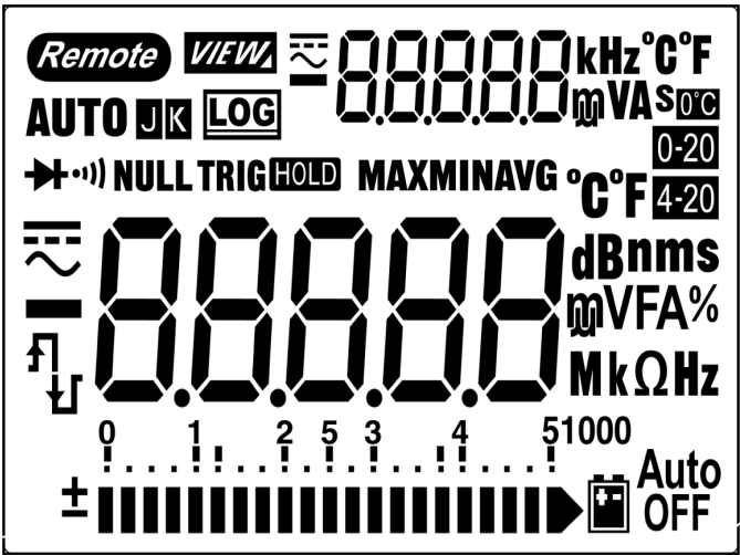
图 6-1 LCD 显示屏
