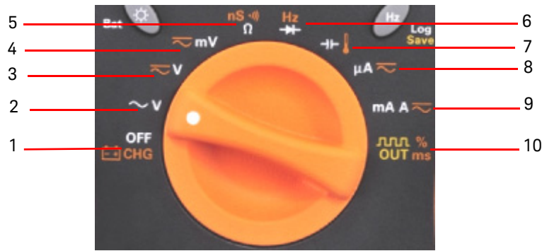
图 1-6 旋转开关
