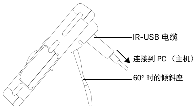
图 1-1 60° 时的倾斜座
