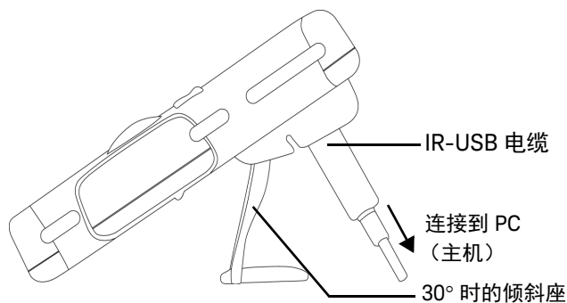
图 1-2 30° 时的倾斜座
