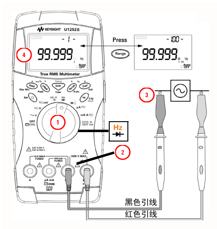
图 2-6 测量频率
