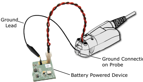
图 45 使用 N2820A 探头在电池供电的设备上进行测量
