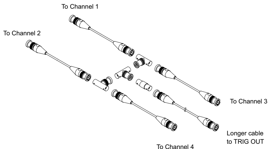
图 50 用于 4 通道示波器的用户校准电缆
