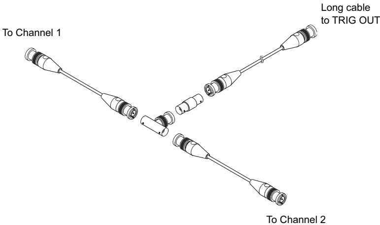
图 49 用于 2 通道示波器的用户校准电缆
