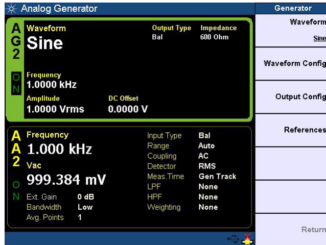
图 10 模拟发生器
