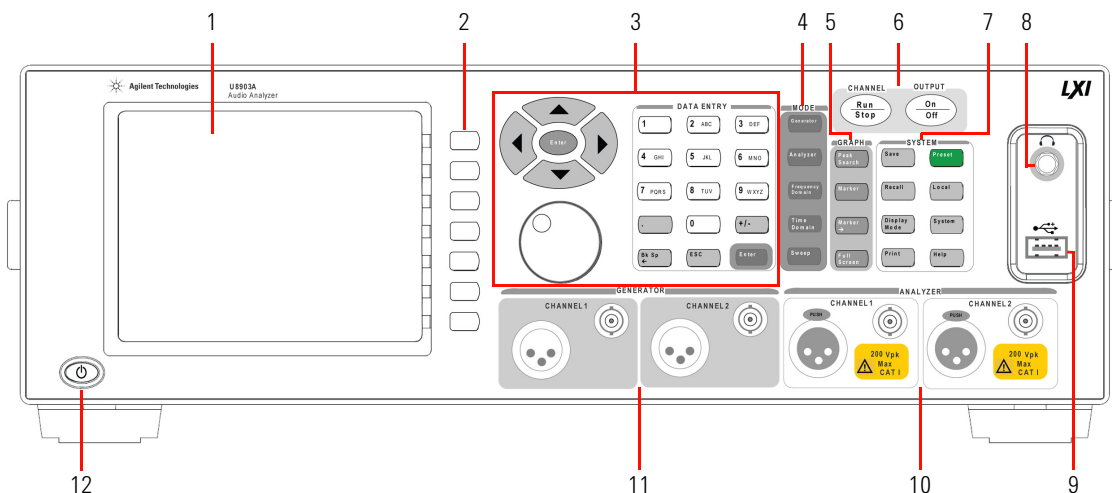
图 1 U8903A 前面板
