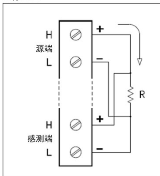
4 线 RTD:
