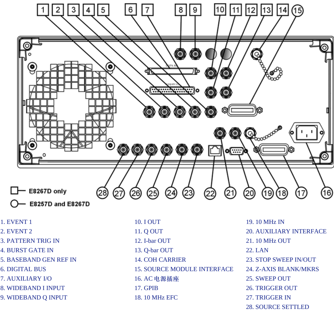
图 1-3 标准后面板示意图
