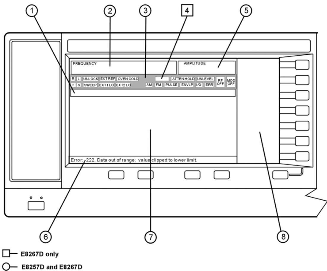
图 1-2 前面板显示屏示意图
