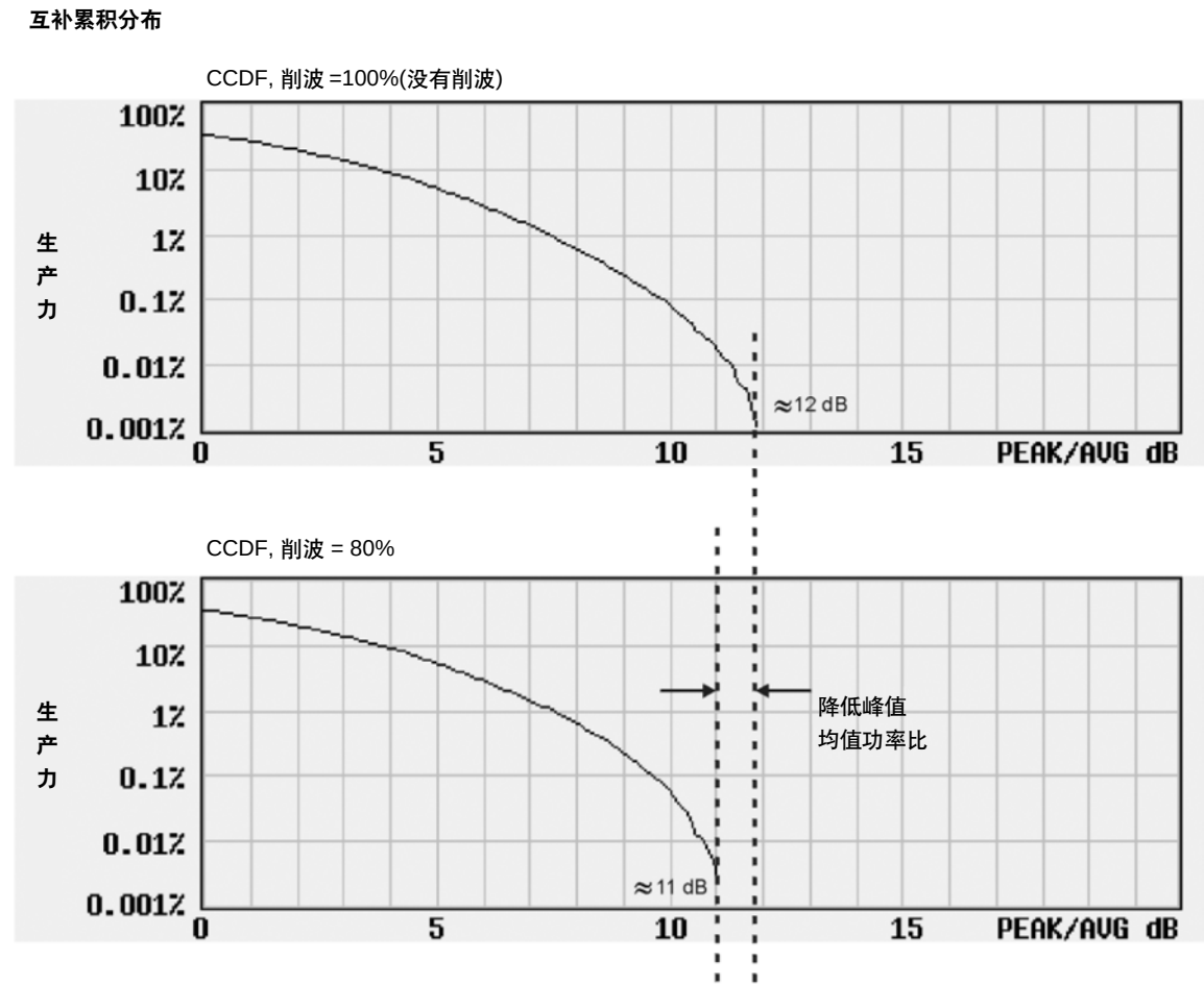
图 3-16 峰值均值功率比
