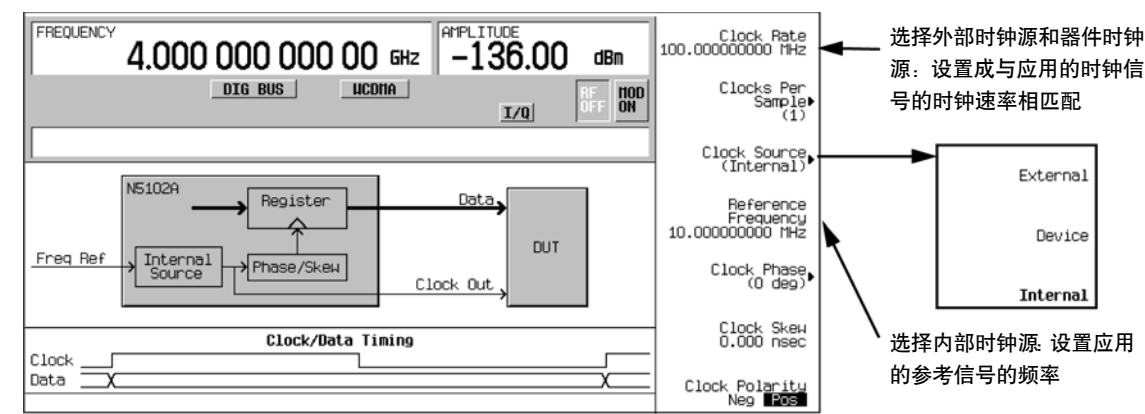
图 11-2 时钟源选择
