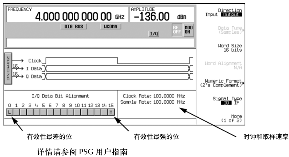
图 11-1 并口配置的数据设置菜单
