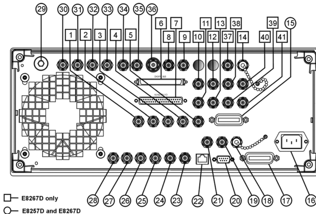
图 1-4 选项 1EM 后面板示意图
