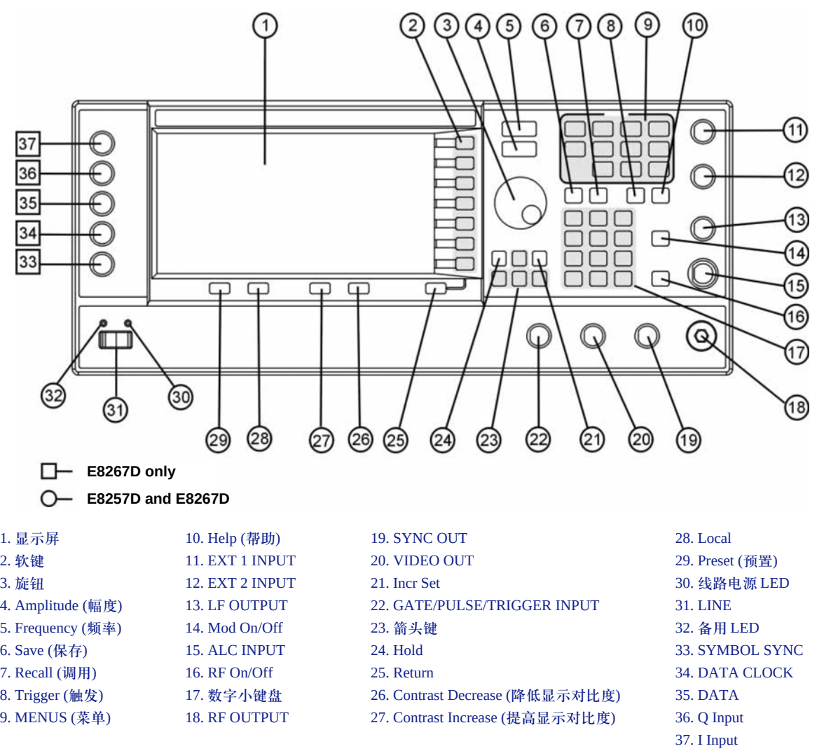
图 1-1 前面板示意图(E8267D PSG 矢量信号源)
