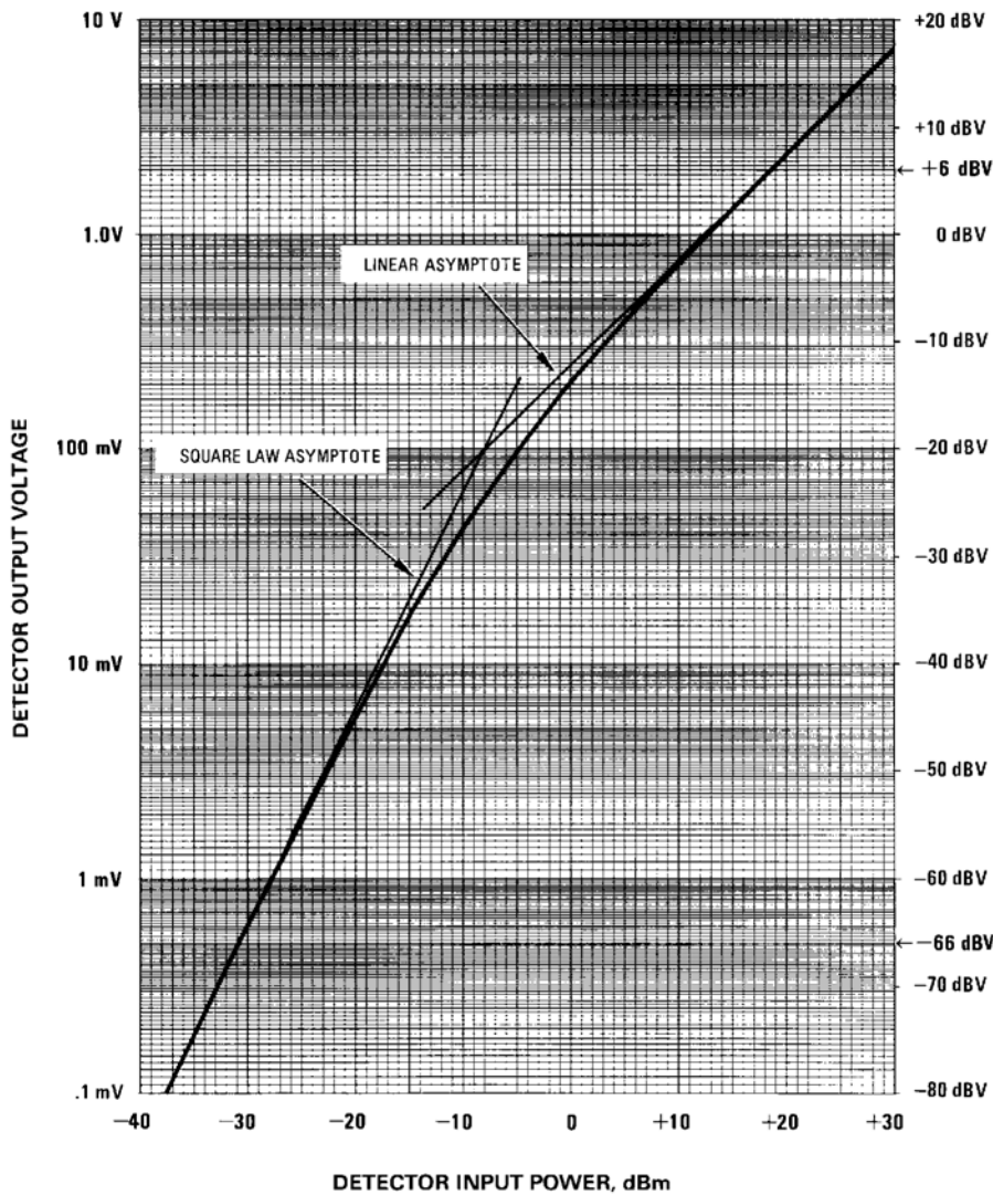
图 4-3 在 25°C 时典型的二极管检测器响应
