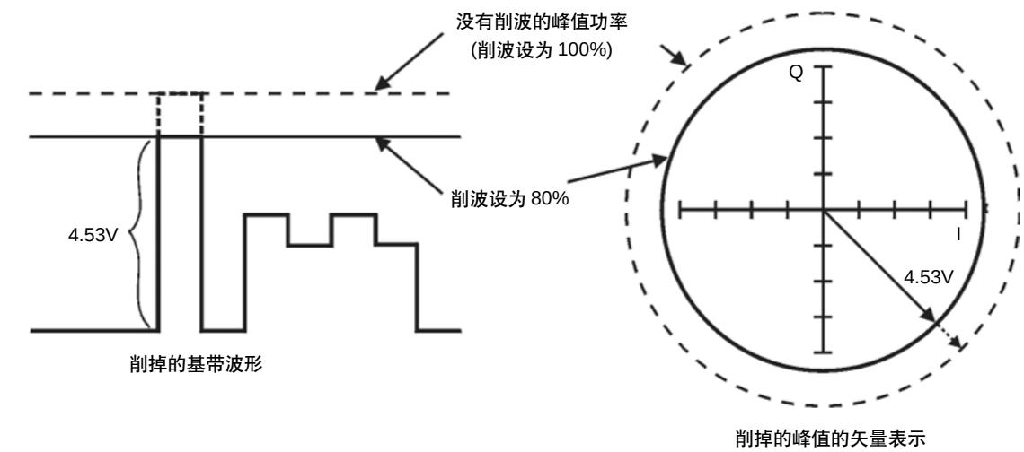
图 3-14 圆形削波
