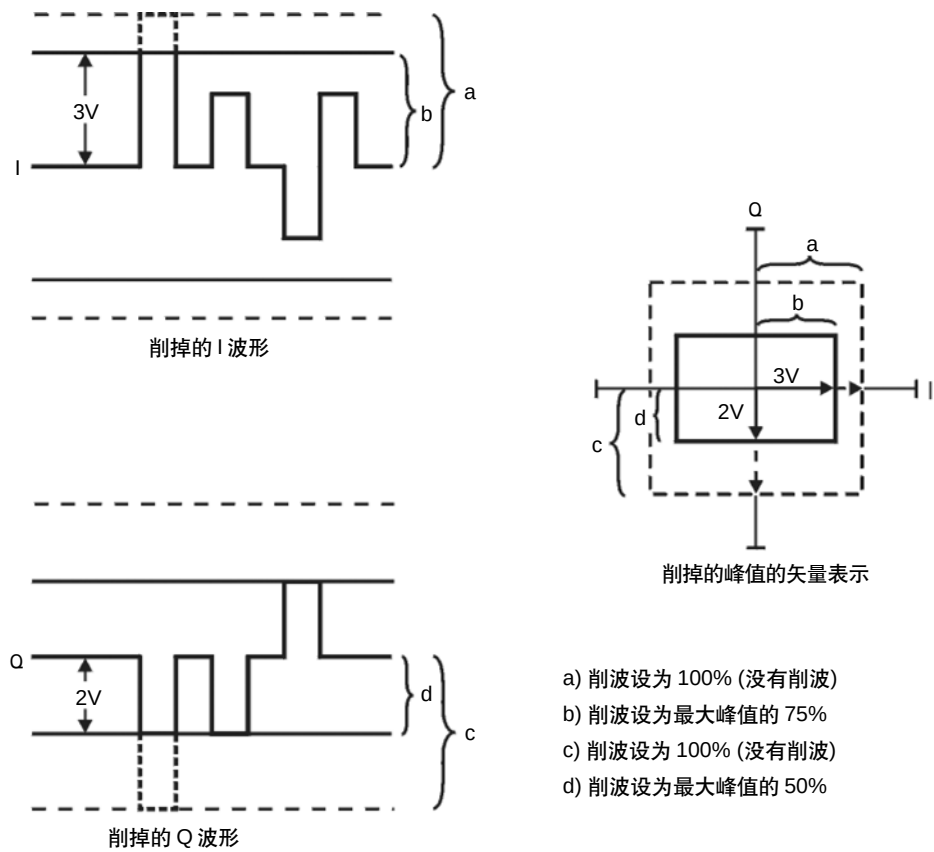
图 3-15 矩形削波
