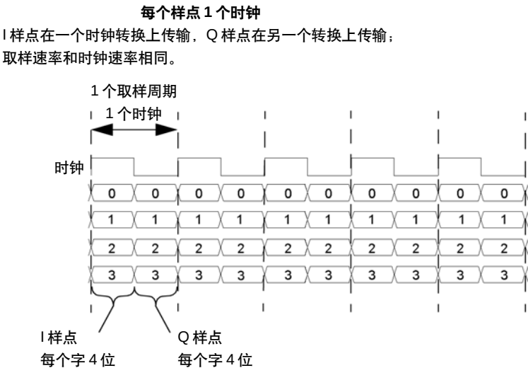
图 11-5 并行 IQ 隔行扫描端口配置的时钟定时
