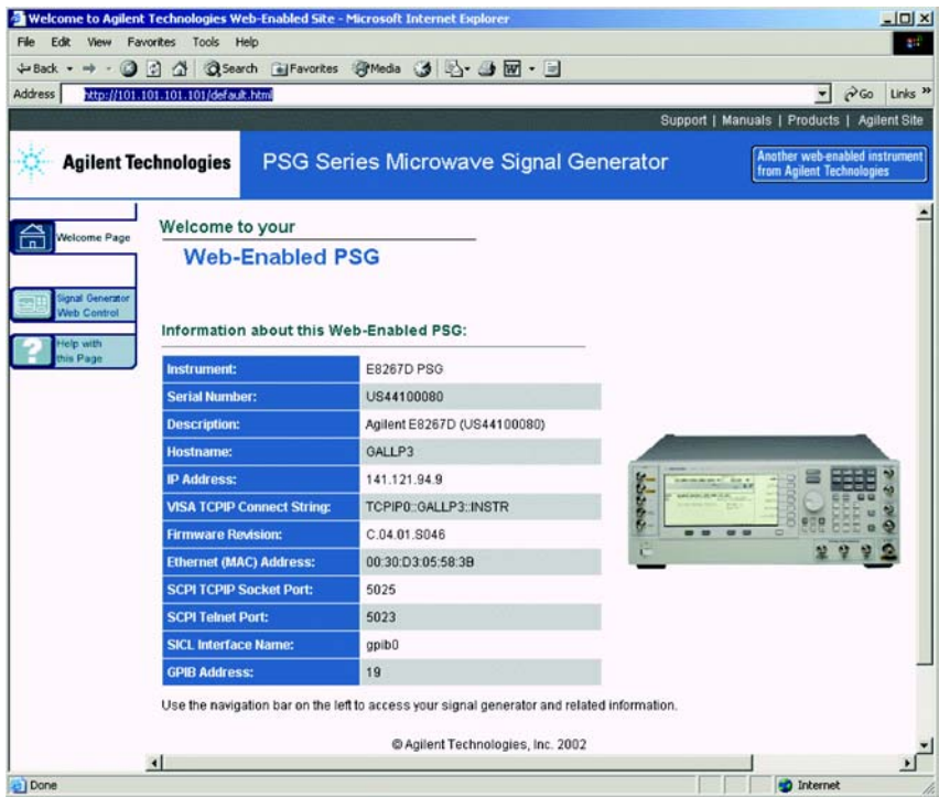
图 2-12 信号源网页
