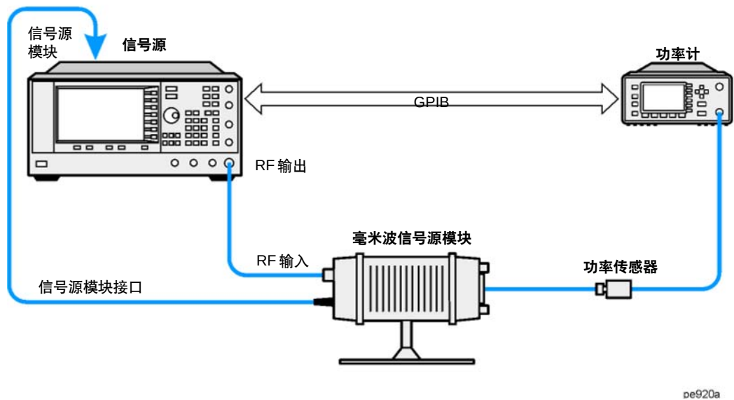
图 4-6 使用毫米波信号源模块和选项 1EA 信号源校正用户平坦度
