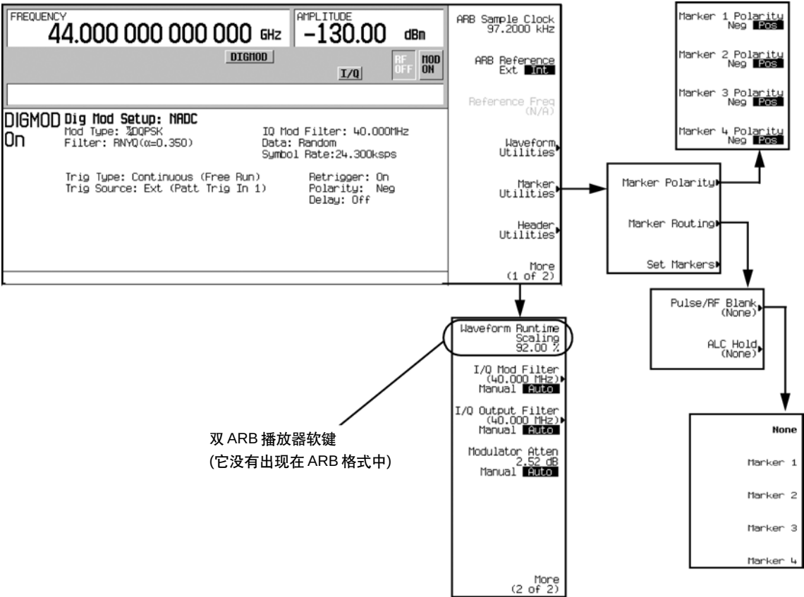
图 3-3 ARB 设置软键菜单和标尺辅助工具
