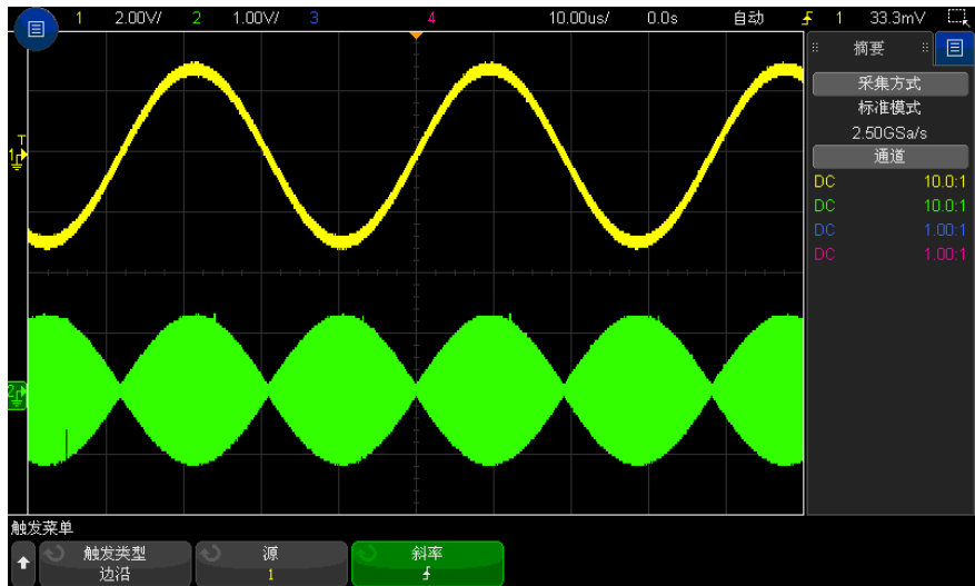
图 27 以 100% 亮度显示的调幅
