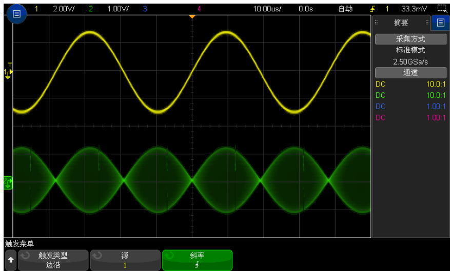
图 28 以 40% 亮度显示的调幅
