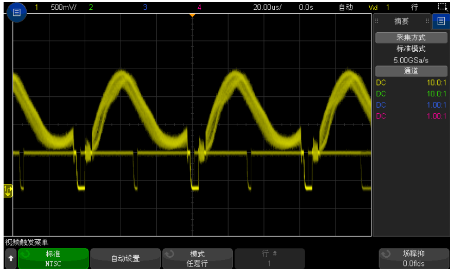
图 30 在所有行上触发
