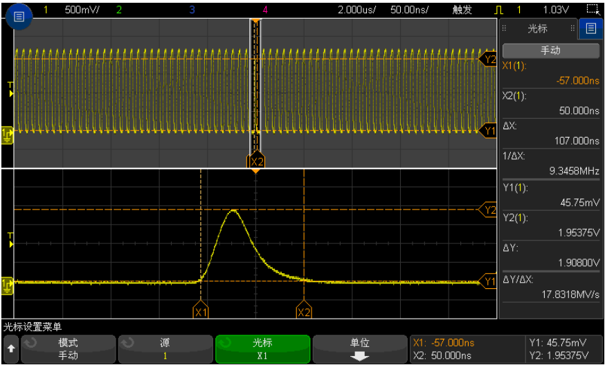
图 44 光标跟踪缩放窗口视图
