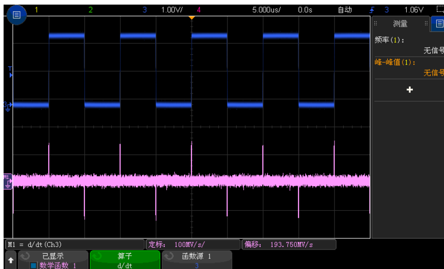
图 8 微分函数示例
