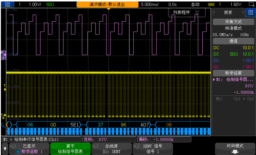
图 21 绘制串行信号图表示例
