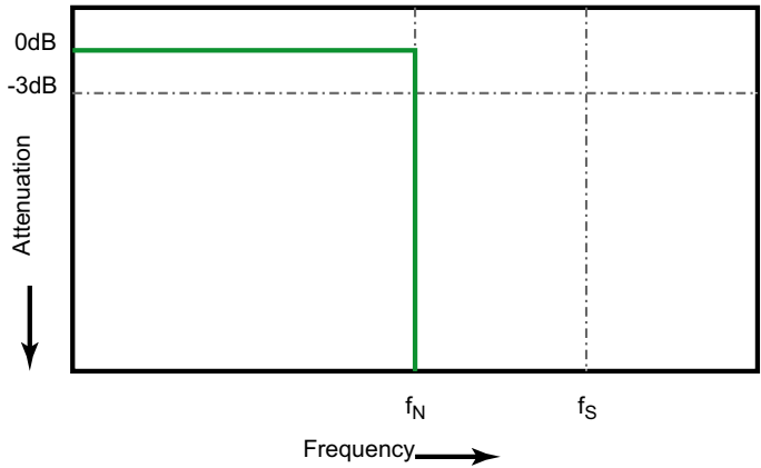
图 36 理论上的砖墙频率响应
