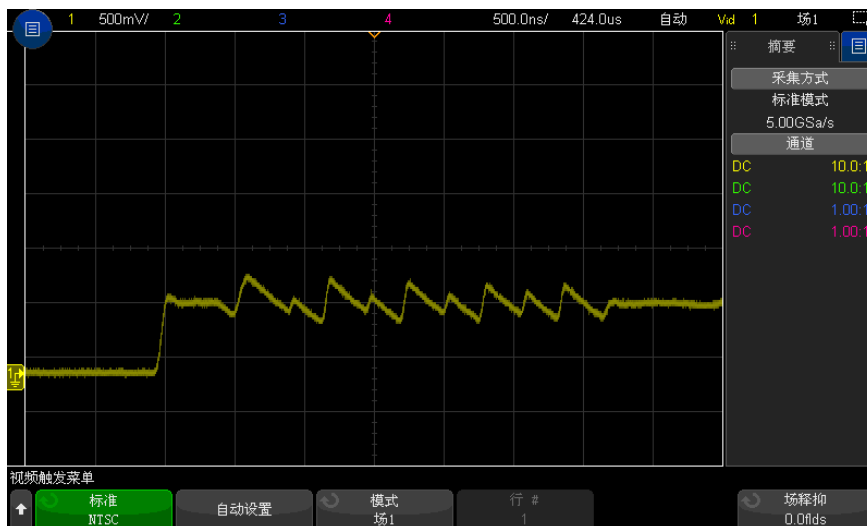
图 33 在彩色场 1 和彩色场 3 上交替触发
