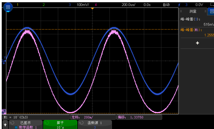
图 15 以 10 为底数的指数示例
