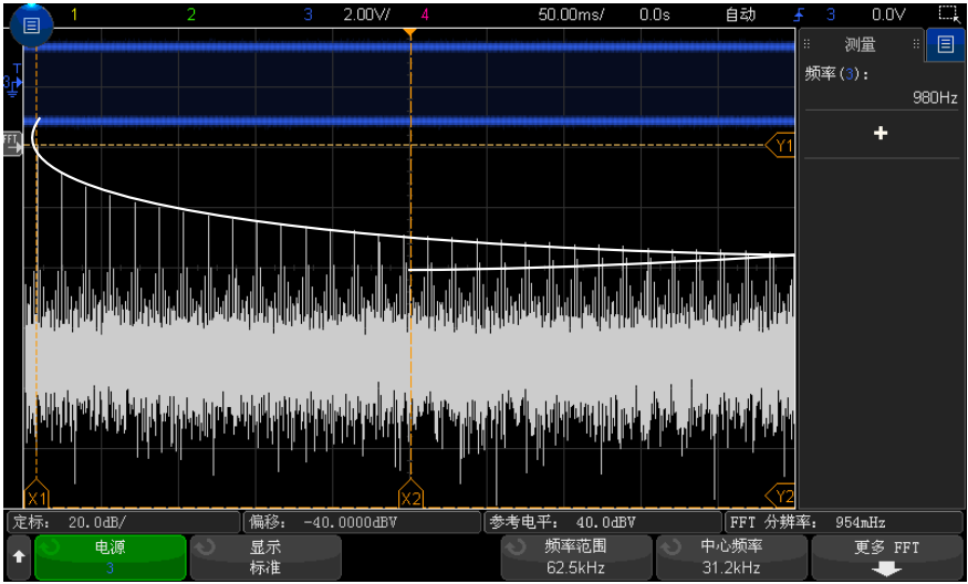
图 5 混叠
