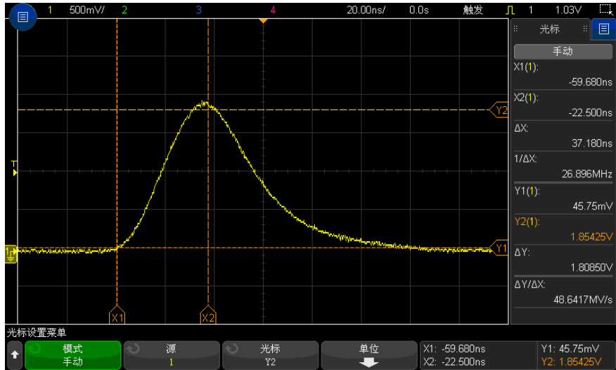
图 42 光标用于测量脉冲宽度而不是测量中阈值点
