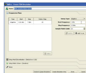
FEM
