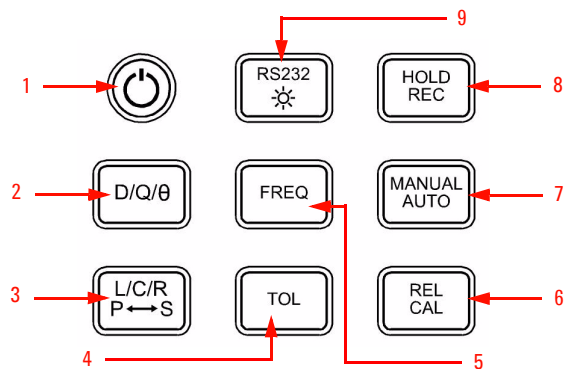
图 1-3 U1731A/U1732A 双显示手持式 LCR 测量仪的键盘
