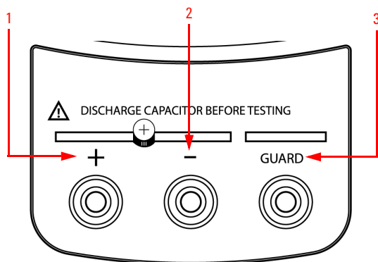
图 1-4 U1731A/U1732A 双显示手持式 LCR 测量仪的输入端子 / 插口
