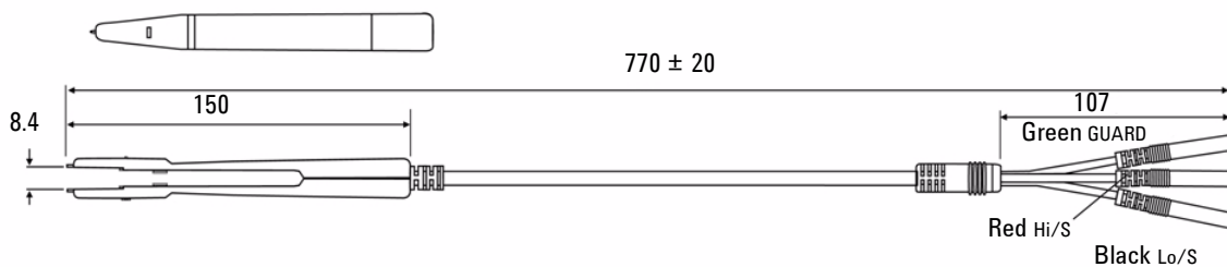
图 4-1 SMD 镊子
