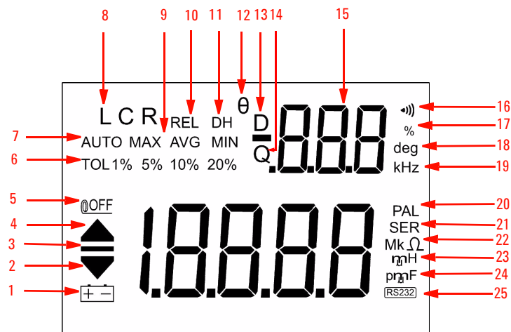
图 1-2 LCD 显示屏
